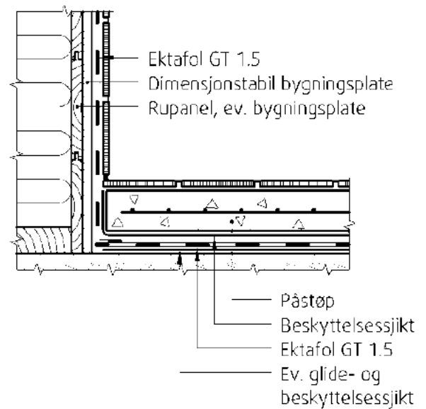
Fig. 6 Ektafol GT 1,5 lagt under påstøp
