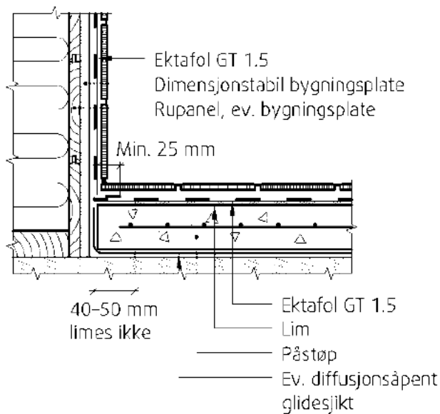
Fig. 5 Ektafol GT 1,5 lagt rett under flisekledning
